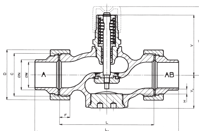
Ventily RV 111 R/W s přivařovacím šroubením
